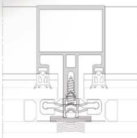
Sección horizontal
